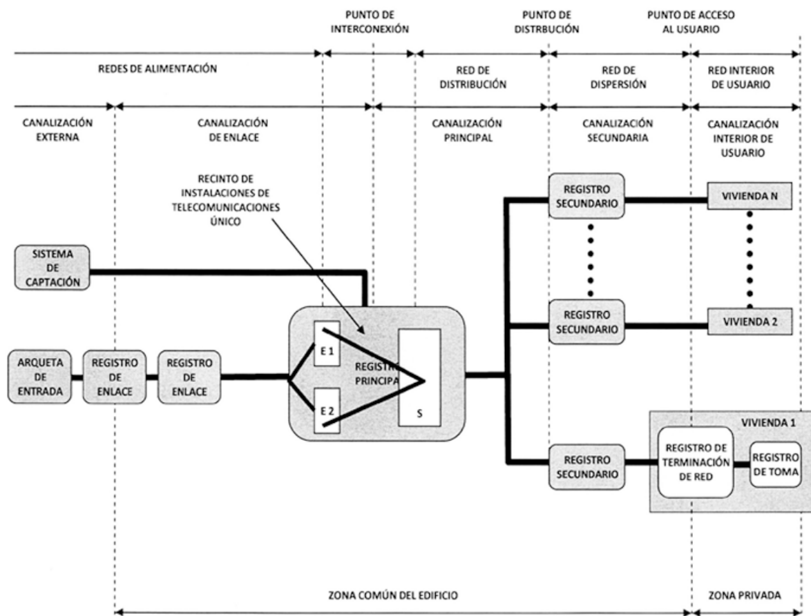
Apéndice 11: Esquema General para agrupaciones de viviendas unifamiliares
