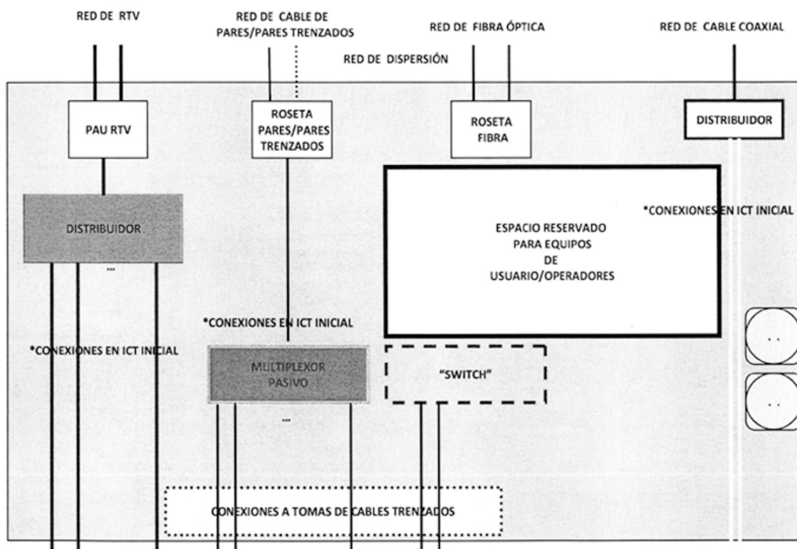
Apéndice 12: Esquema General de Ubicación de Elementos en Registro de Terminación de Red
