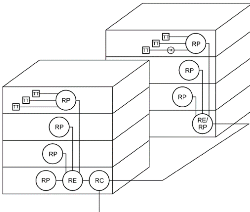
Distribución de la Red de Cableado Estructurado por edificios y por plantas
