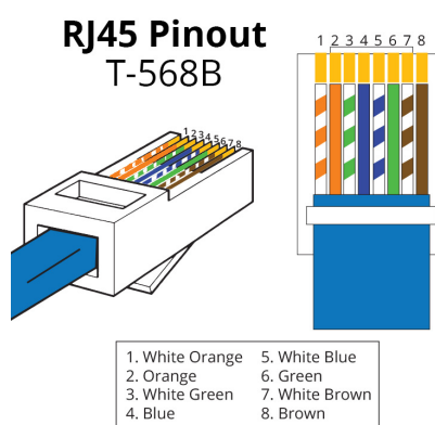
Figura: Esquema de conexionado Norma EIA/TIA 568 B.
