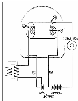
Moderno triodo
