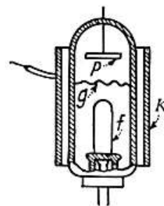
Válvula Weagant de cuatro elementos. P = Placa, f = filamento, g = rejilla interior, K = anillo exterior
