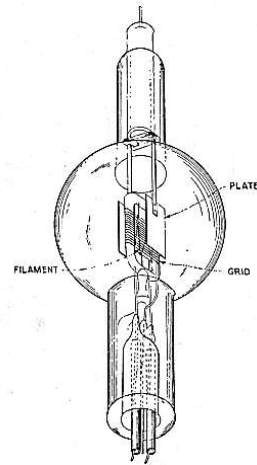
El Piotron.
