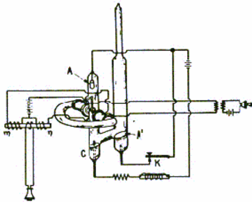
Amplificador de vapor de mercurio de H. D. Arnold
