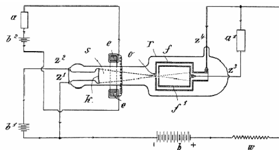
Primer tubo amplificador de rayos catódicos de Robert von Lieben (Pat. DRP 179807)
