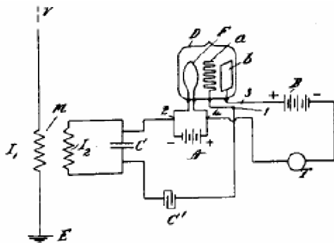
El Audión DeForest
