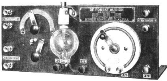
Receptor audión RJ9 DeForest con sus potenciómetros de ajuste
