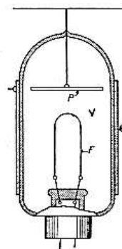
Válvula Weagant de control externo.
