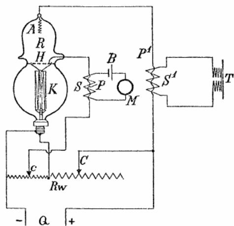
Patente DRP249142. Controla el flujo de corriente entre el cátodo y el ánodo por medio del disco perforado (rejilla) H
