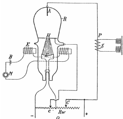
Patente DRP249142. Por medio de la bobina E se controla el flujo de corriente entre el cátodo y el ánodo
