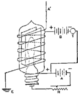
Detector con control magnético externo.
