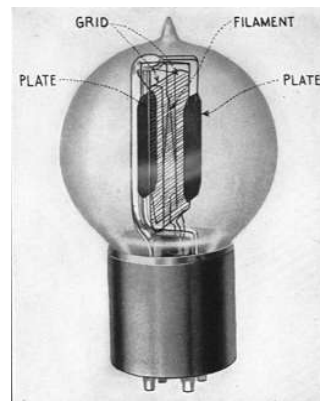
Fotografía de un Piotron.
