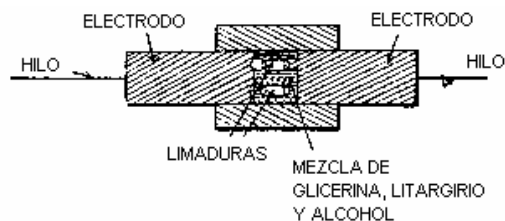
El “go-responder” DeForest
