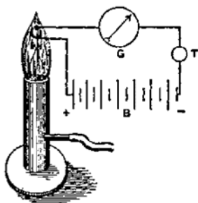
El detector de llama DeForest
