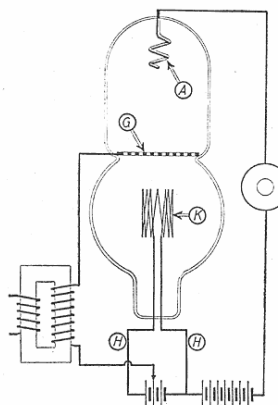
Válvula Lieben definitiva Pat. DRP 254588. El interior está lleno de vapor de mercurio a baja presión
