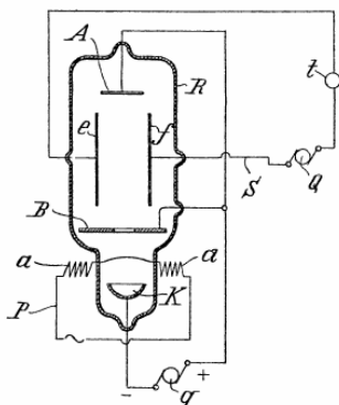
Patente DRP236716. Controla la ionización del gas interior para variar la corriente que circula entre las placas e y f
