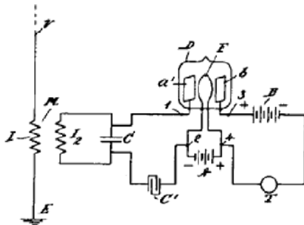
El "diodo de doble placa" DeForest.
