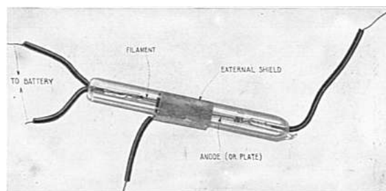
Válvula Weagant de control externo.
