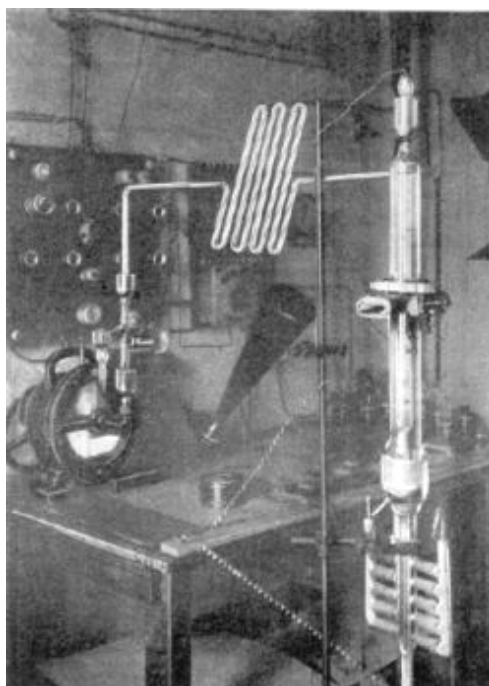
Primer tubo amplificador de rayos catódicos de von Lieben
